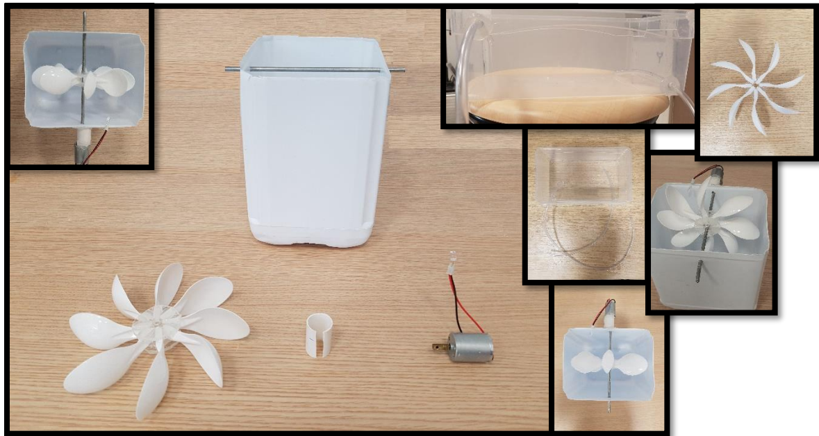
Şekil 5-4 Su gücünden faydalanan elektrik enerjisi elde etmek için deney elemanları ve düzeneği
