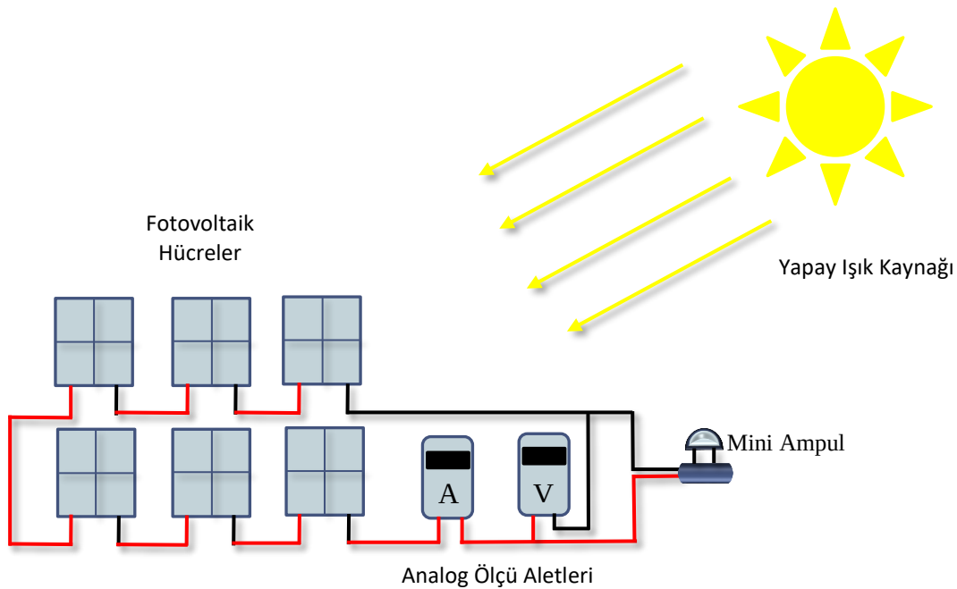
Şekil 7-2 PV hücrelerin seri ve paralel bağlaması etkinliği
