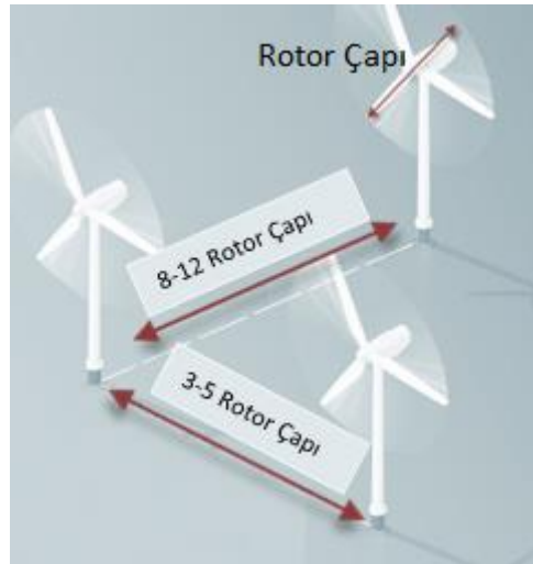
Şekil 9-10 Yatay eksenli rüzgâr türbinlerini yerleştirilmesi
