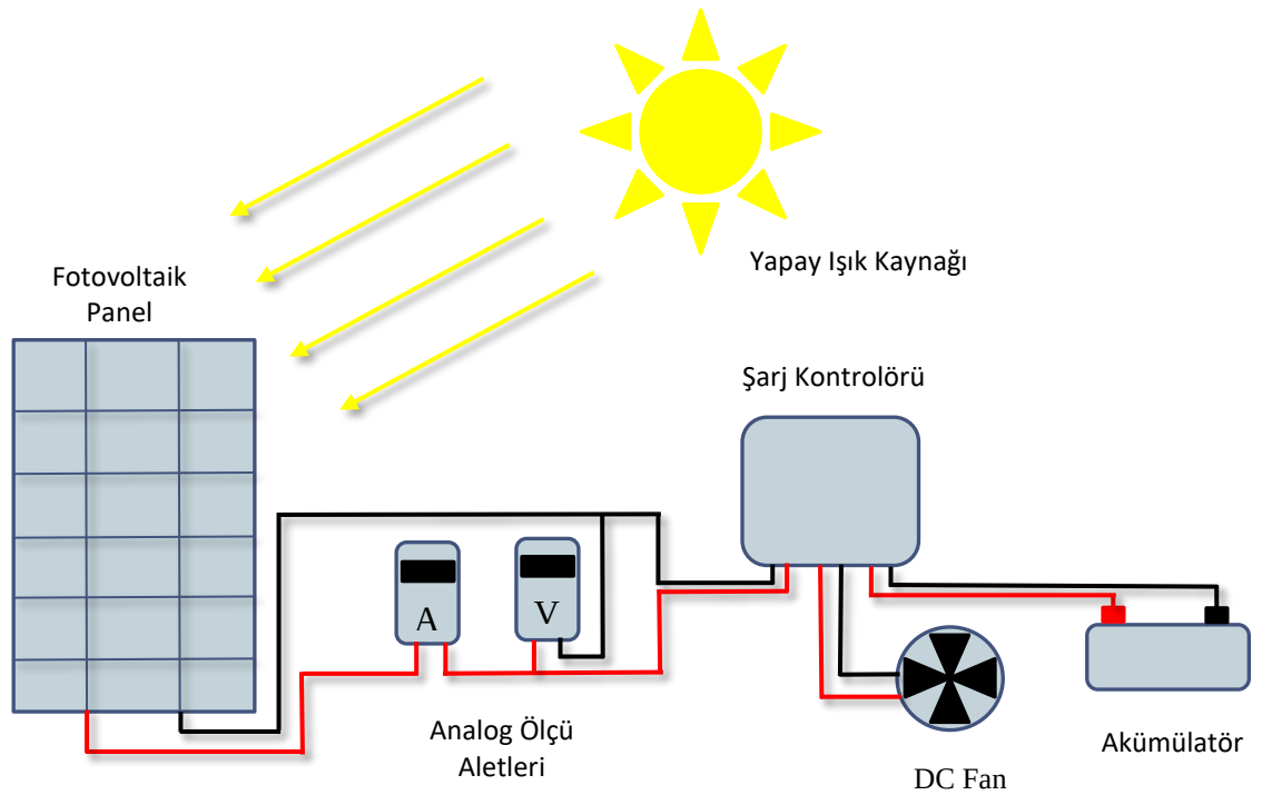
Şekil 7-4 PV panelin DC yükü beslemesi ve batarya şarjı etkinliği
