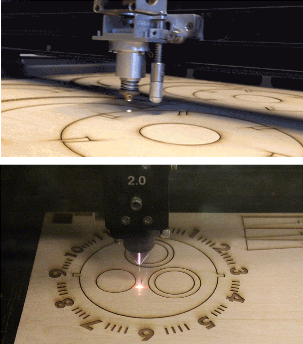
Şekil 1.15. Lazer kesim/markalama temel prensibi (kaynak: üst: https://gifer.com/en/FNu5 , alt: https://www.alexsg.com/portfolio/clockwork-chair/ )
