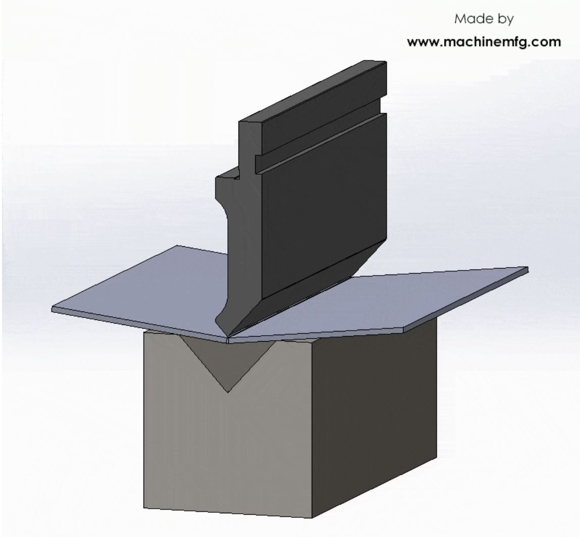
Şekil 1.12. Sac büküm temel prensibi (kaynak: https://medium.com/@ishane1112/press-brake-the-ultimate-guide-a31ffe08027 )
